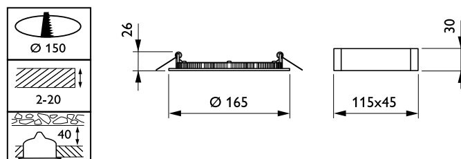
1.000 lm indbygget / påbygget
