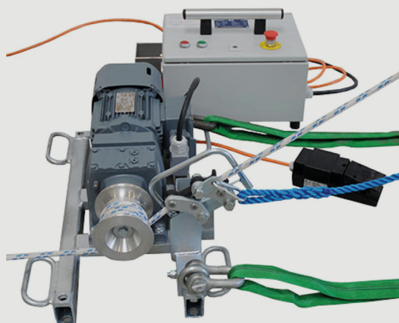
Træktov Dobbeltflettet polyesterreb med to splejsede løkker (en i hver ende).
