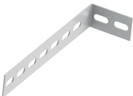
90° vinkelbeslag (H: 37 mm)
